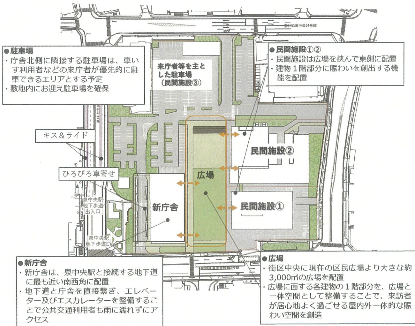
〈図 配置図〉
